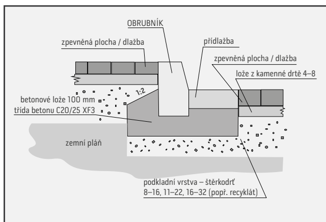
Schematické vyobrazenie usadzovania obrubníka a príďlažby
