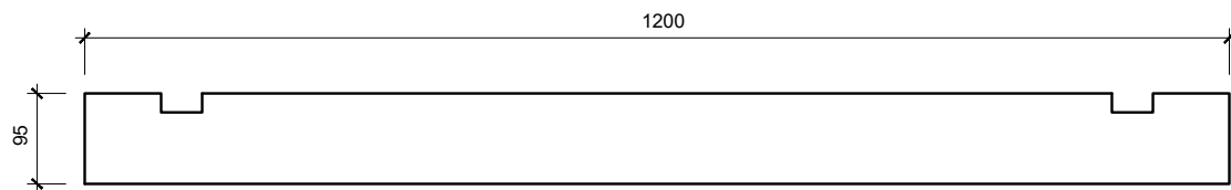
PŮDORYS ukončující prvek
