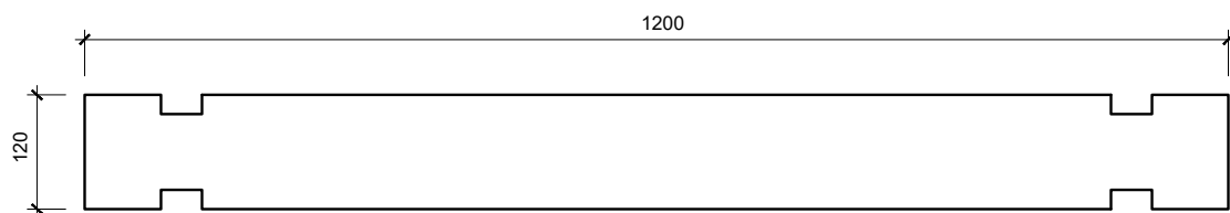
PŮDORYS základní prvek
