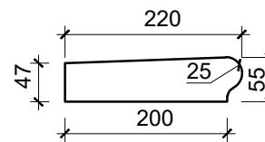
OBLOUK R 1,45 PUL
