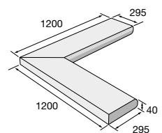
BL 120/30/4 VR S – vnitřní roh sestava
