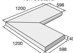
BL 120/60/4 VR S – vnitřní roh sestava
