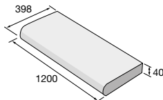
BL 120/40/4 PR – průběžný
