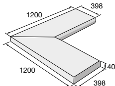
BL 120/40/4 VR S – vnitřní roh sestava
