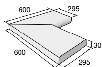
BL 60/30/3 VR S – vnitřní roh sestava
