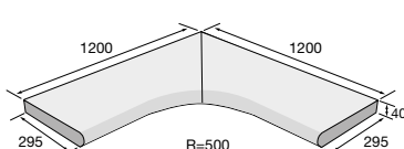
BL 120/30/4 VR S R 0,5 – vnitřní roh sestava
