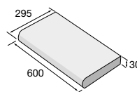
BL 60/30/3 PR – průběžný
